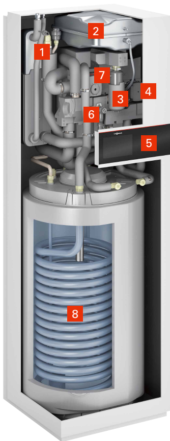
VITOCAL 222-S ar vienu apsildes/dzesēšanas loku
