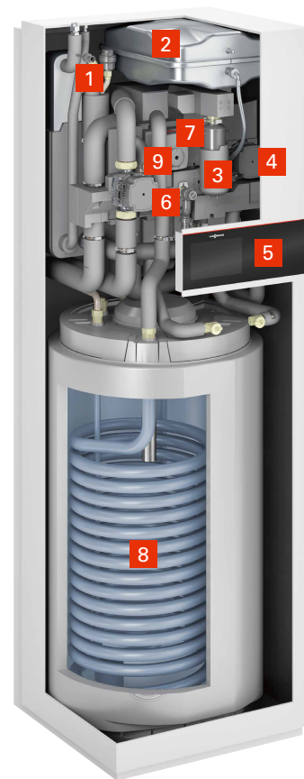
VITOCAL 222-S ar diviem apsildes/dzesēšanas lokiem
