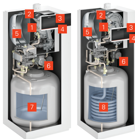
Vitodens 222-F ar emaljētu akumulācijas tvertni (tips B2TE)
